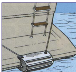
Parabordo in PVC gonfiabile per poppa di barche a vela, per protezione plancette poppiere e per protezione ruota di prua. Inflatable fender for sail boat transom, to protect stern or bow.
